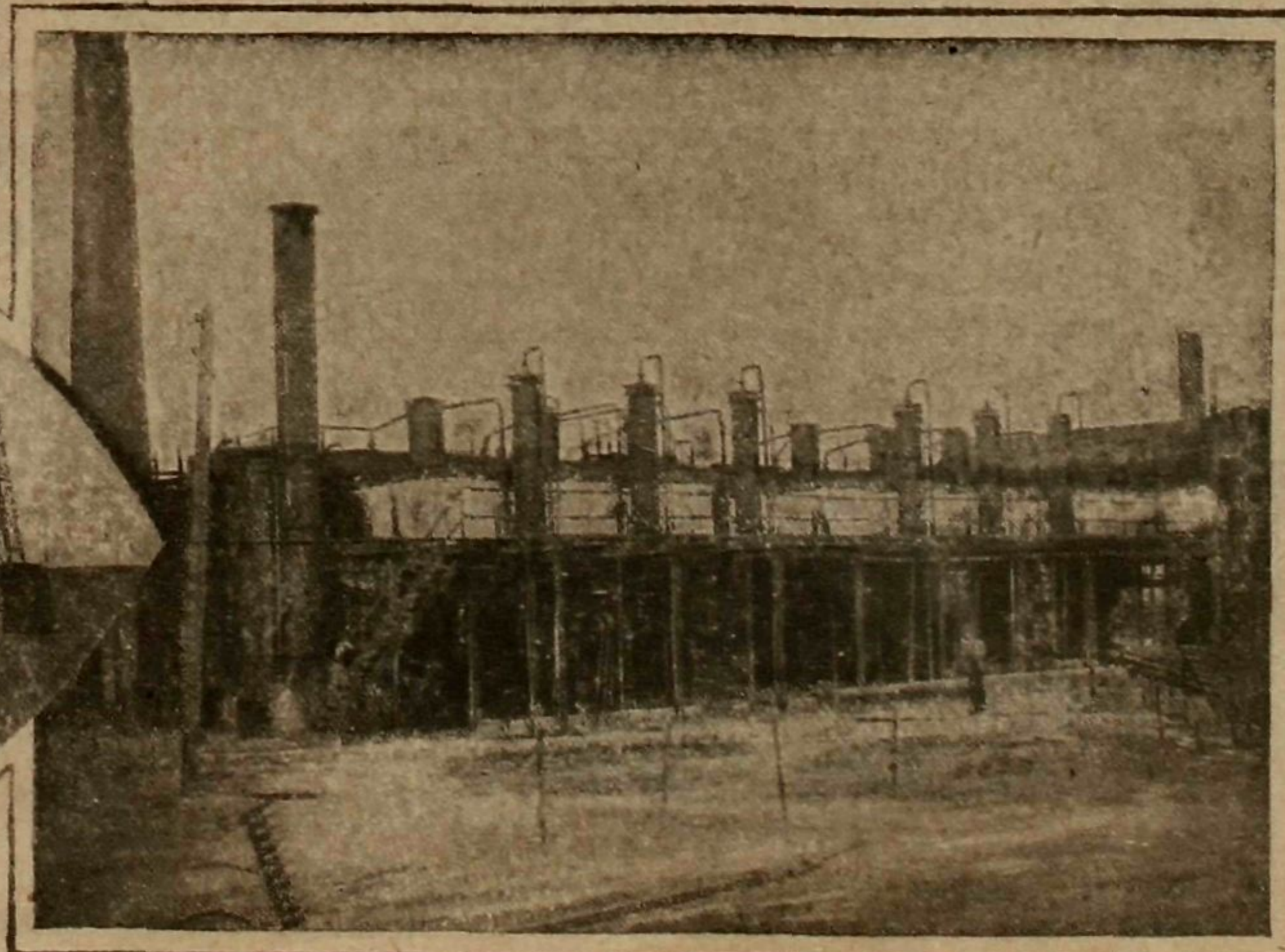
Сверху вниз изображено: 1) Старо-Грозненские промысла; 2) станция для заполнения цистерн нефтью; 3) фонтанирующая нефтяная скважина, нижняя часть вышки; 4) нефтяные склады—цистерны; и 5) завод для очистки от нефти парафина.
